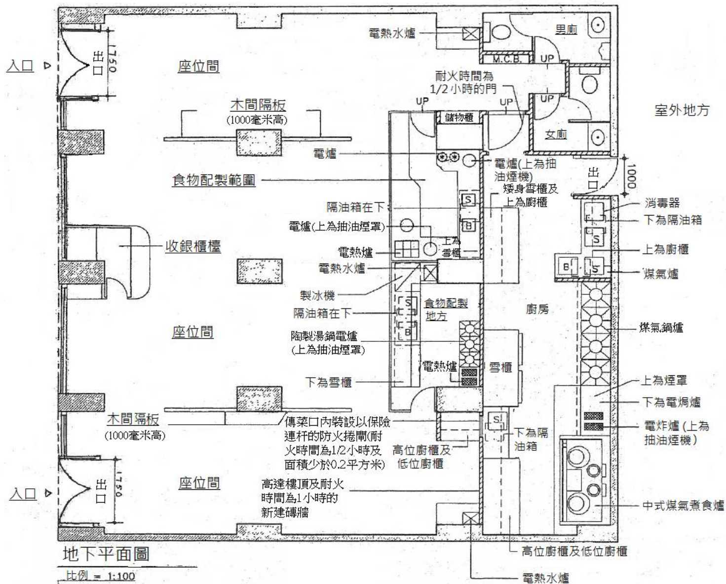
設計圖則 (樣本二)
