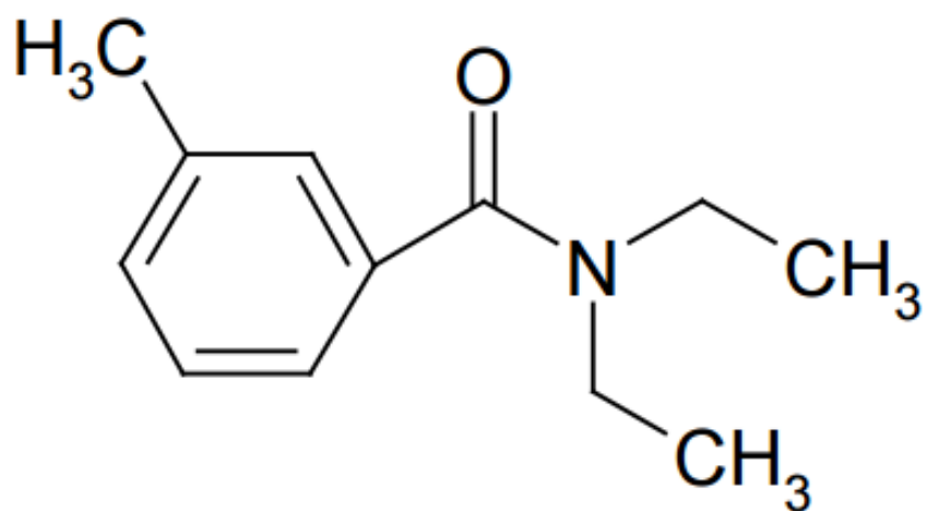
图一：N,N-Diethyl-3-methylbenzamide，避蚊胺的化学结构。
