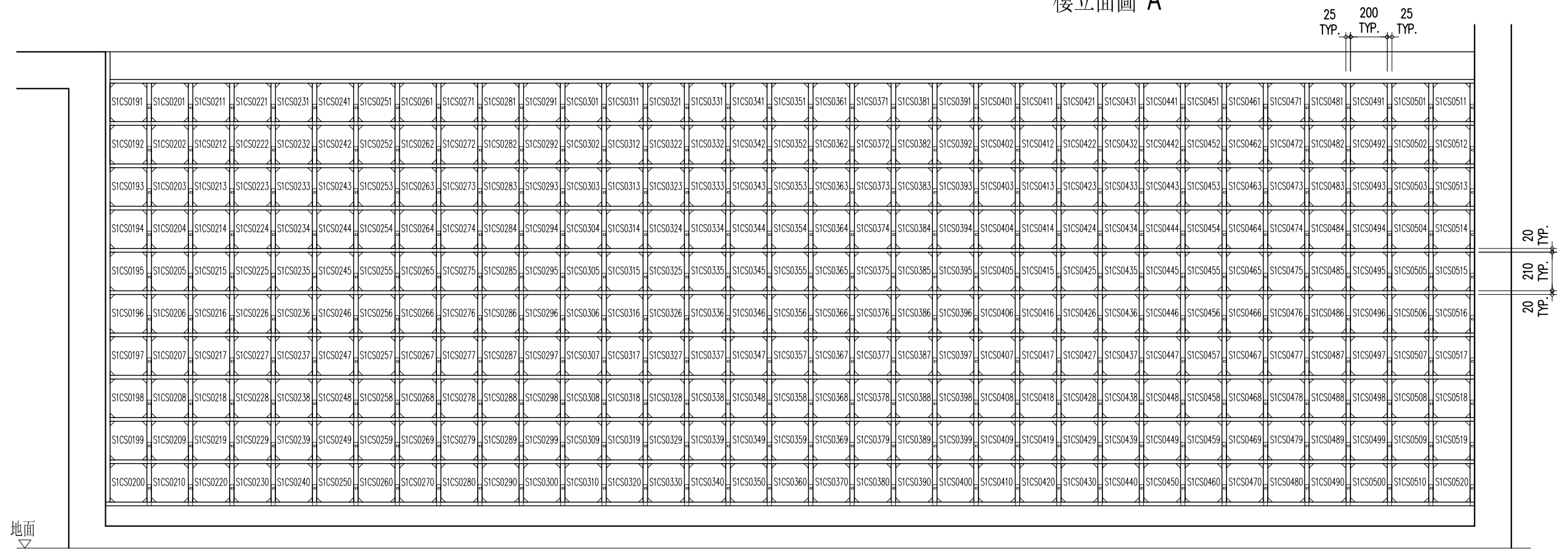
SICS0001 ~ SICS0190 一樓立面圖 A
