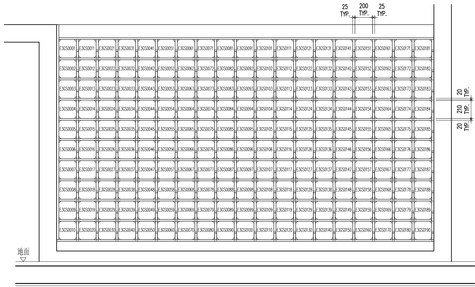
E3GS0001~E3GS0190 三樓立面圖 A
