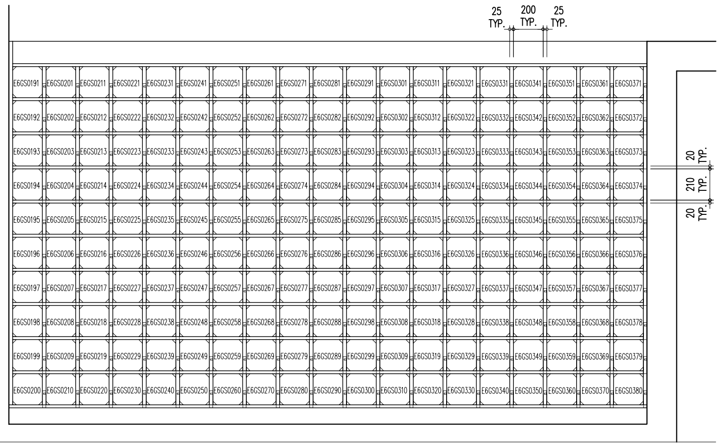
E6GS0191~ E6GS0380 六樓立面圖 A
