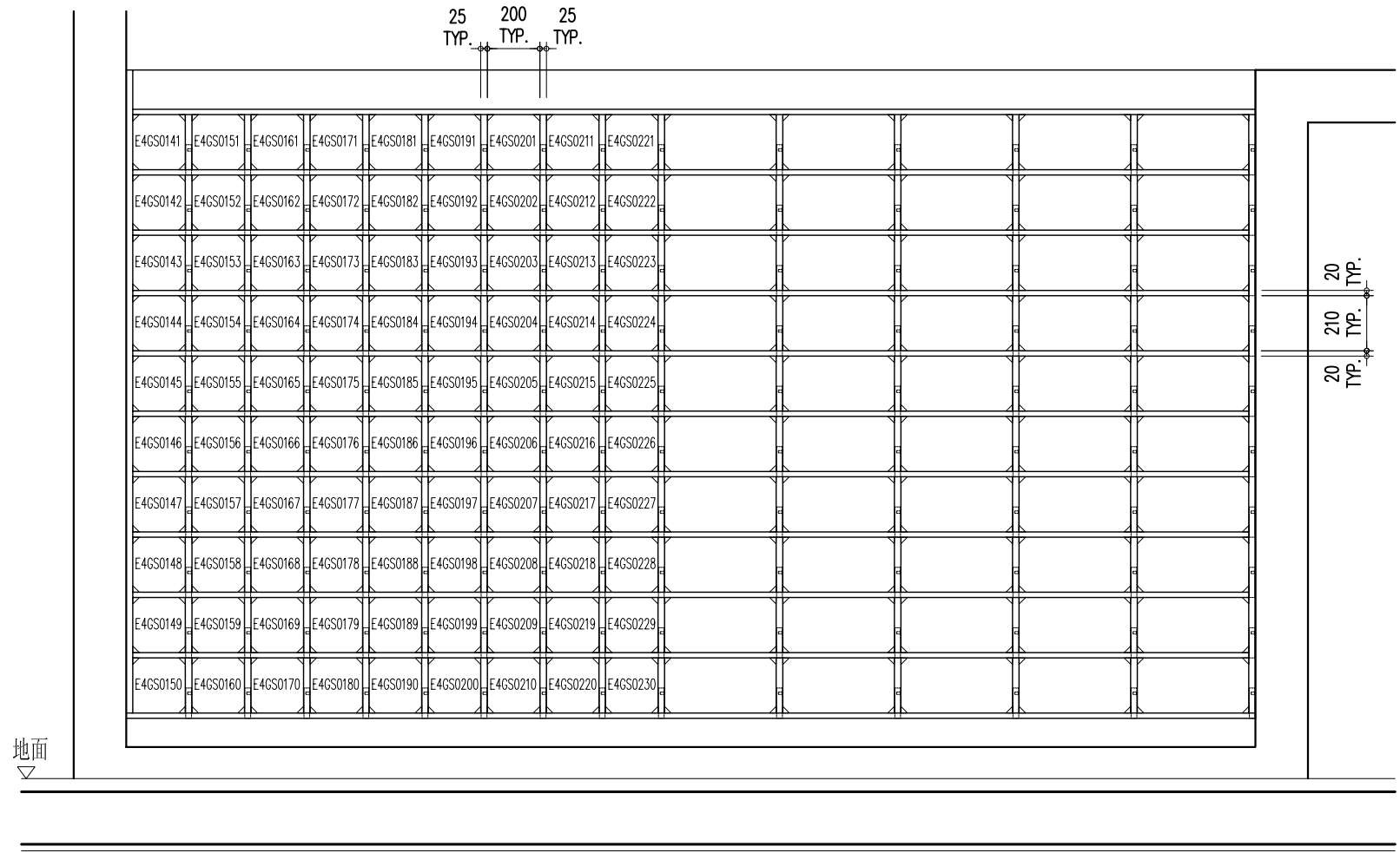
E4GS0141 ~ E4GS0230 四樓立面圖 A
