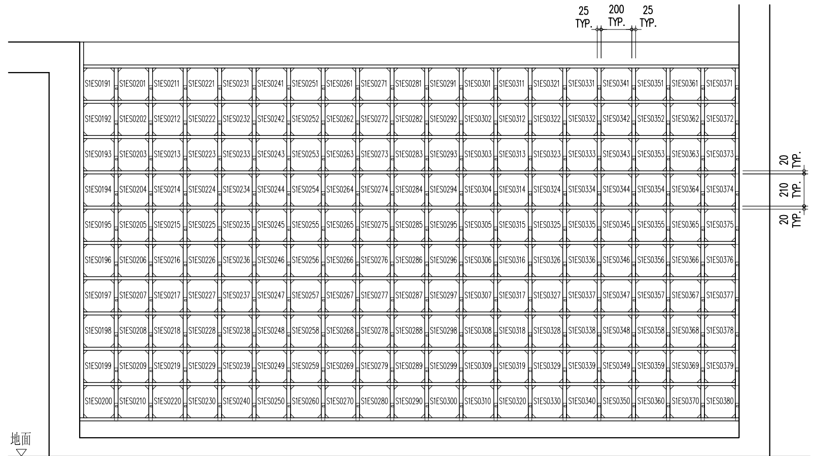
S1ES0191 ~ S1ES0380 一樓立面圖 A
