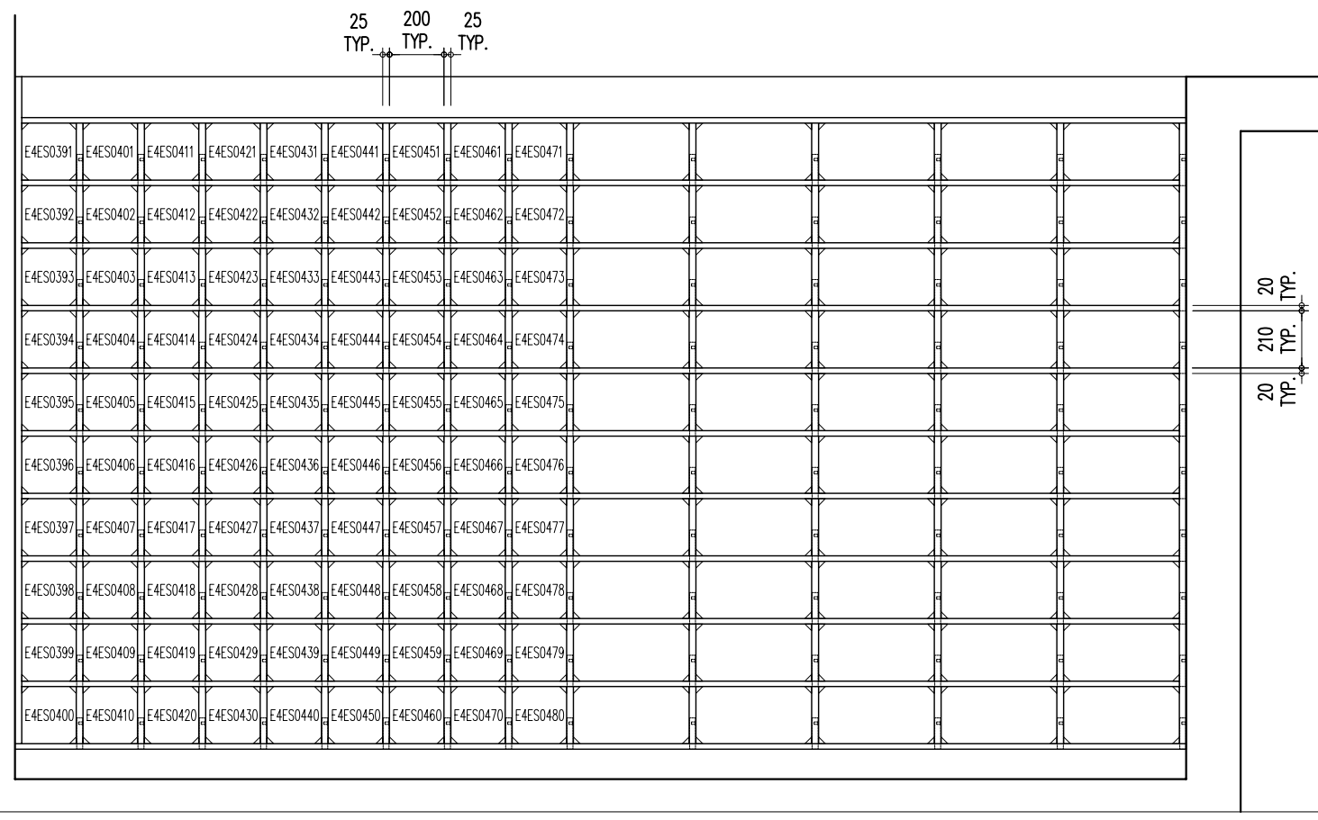
E4ES0391 ~ E4ES0480 四樓立面圖 A
