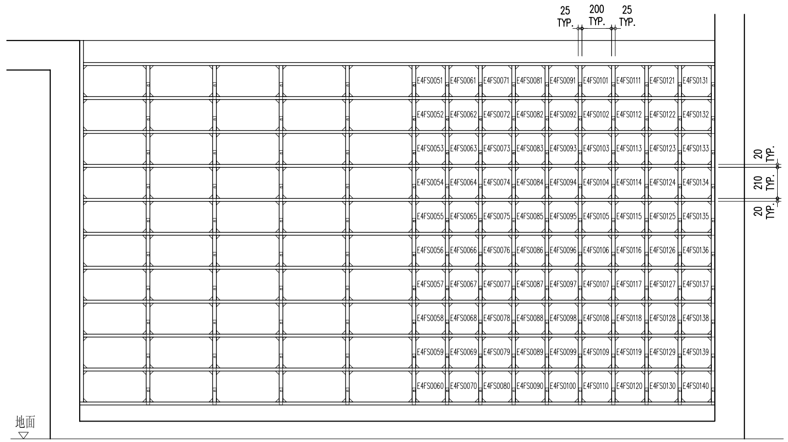
E4FS0051 ~ E4FS0140 四樓立面圖 A
