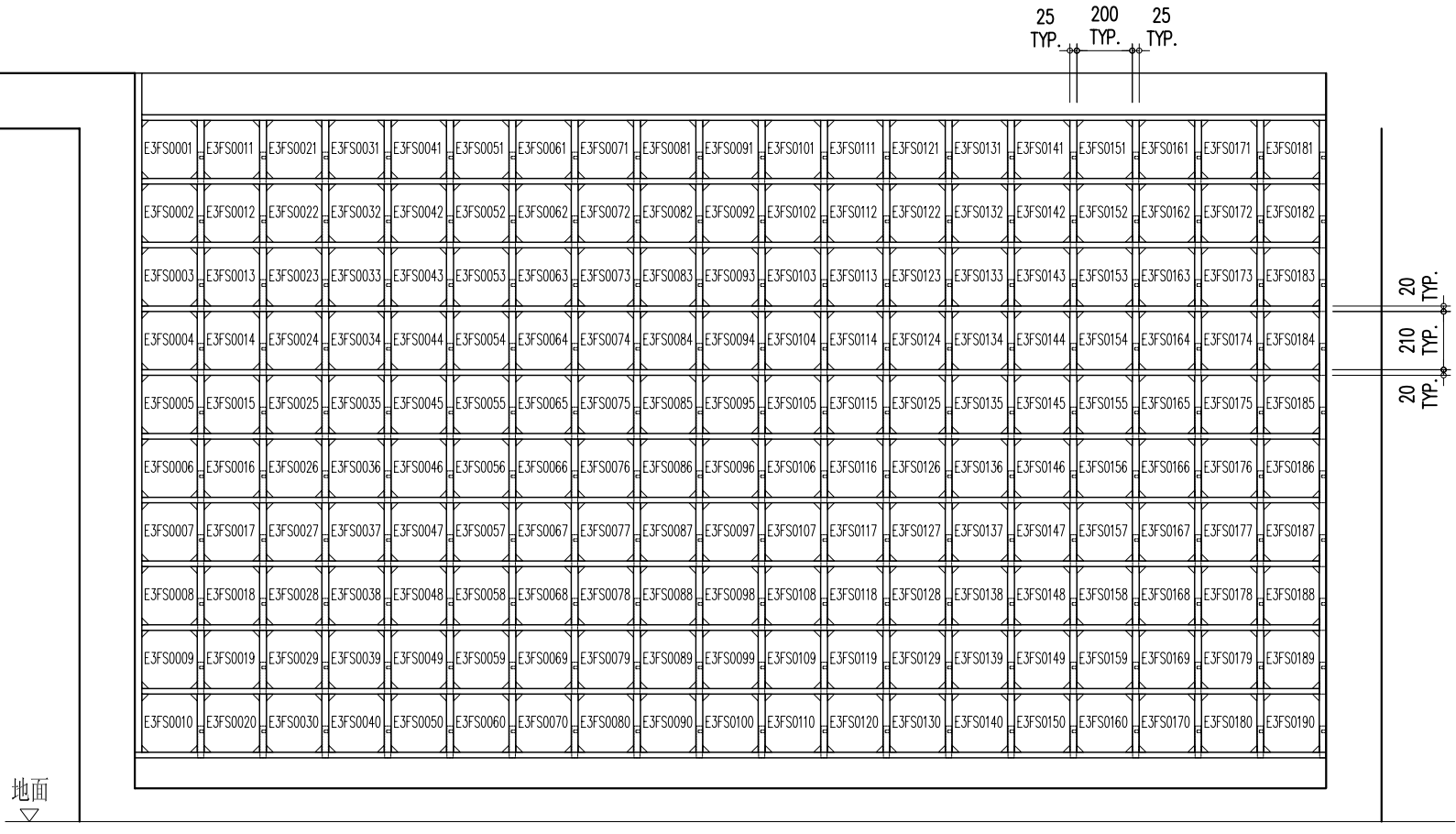
E3FS0001 ~ E3FS0190 三樓立面圖 A
