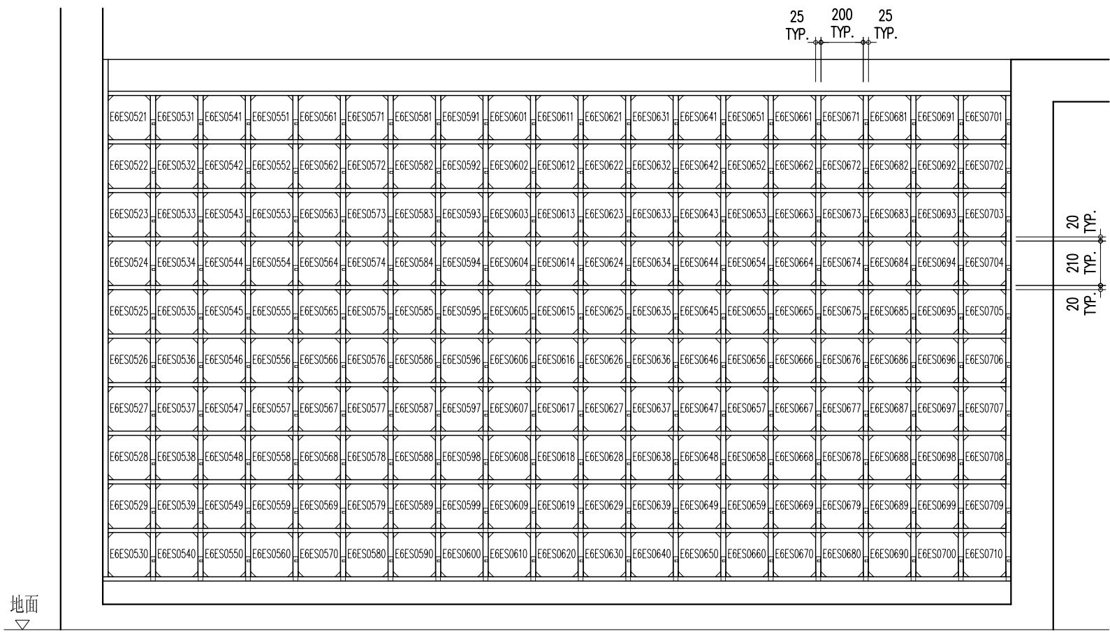
E6ES0521 ~ E6ES0710 六樓立面圖 A
