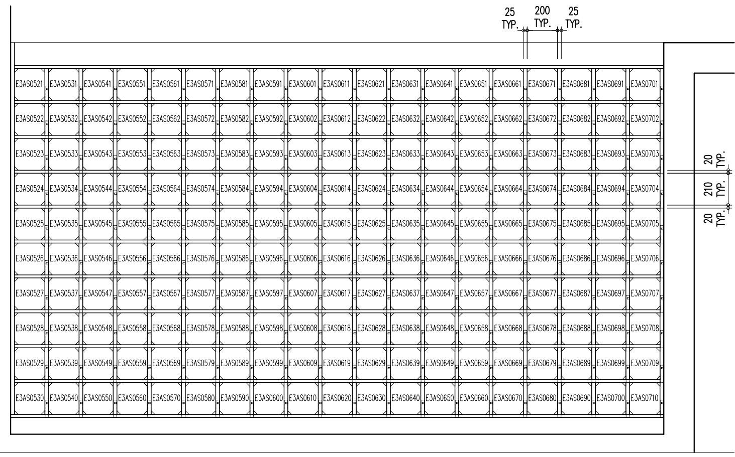
E3AS0521 ~ E3AS0710 三樓立面圖 A
