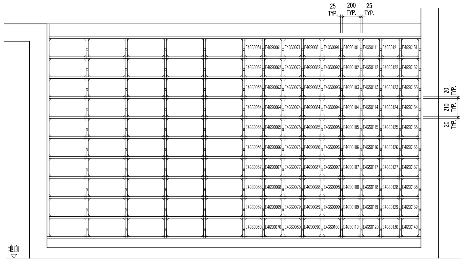
E4GS0051 ~ E4GS0140 四樓立面圖 A
