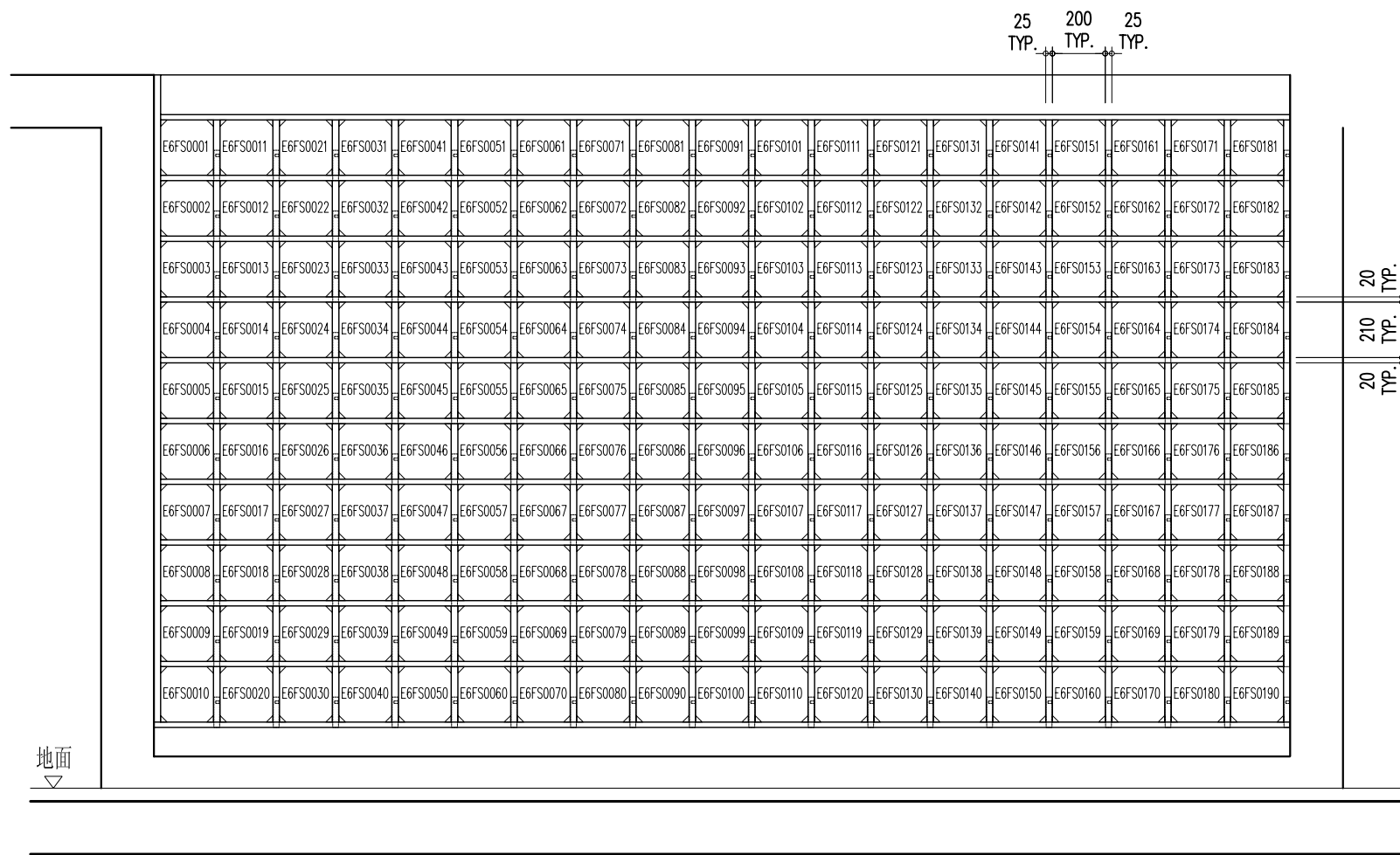
E6FS0001 ~ E6FS0190 六樓立面圖 A
