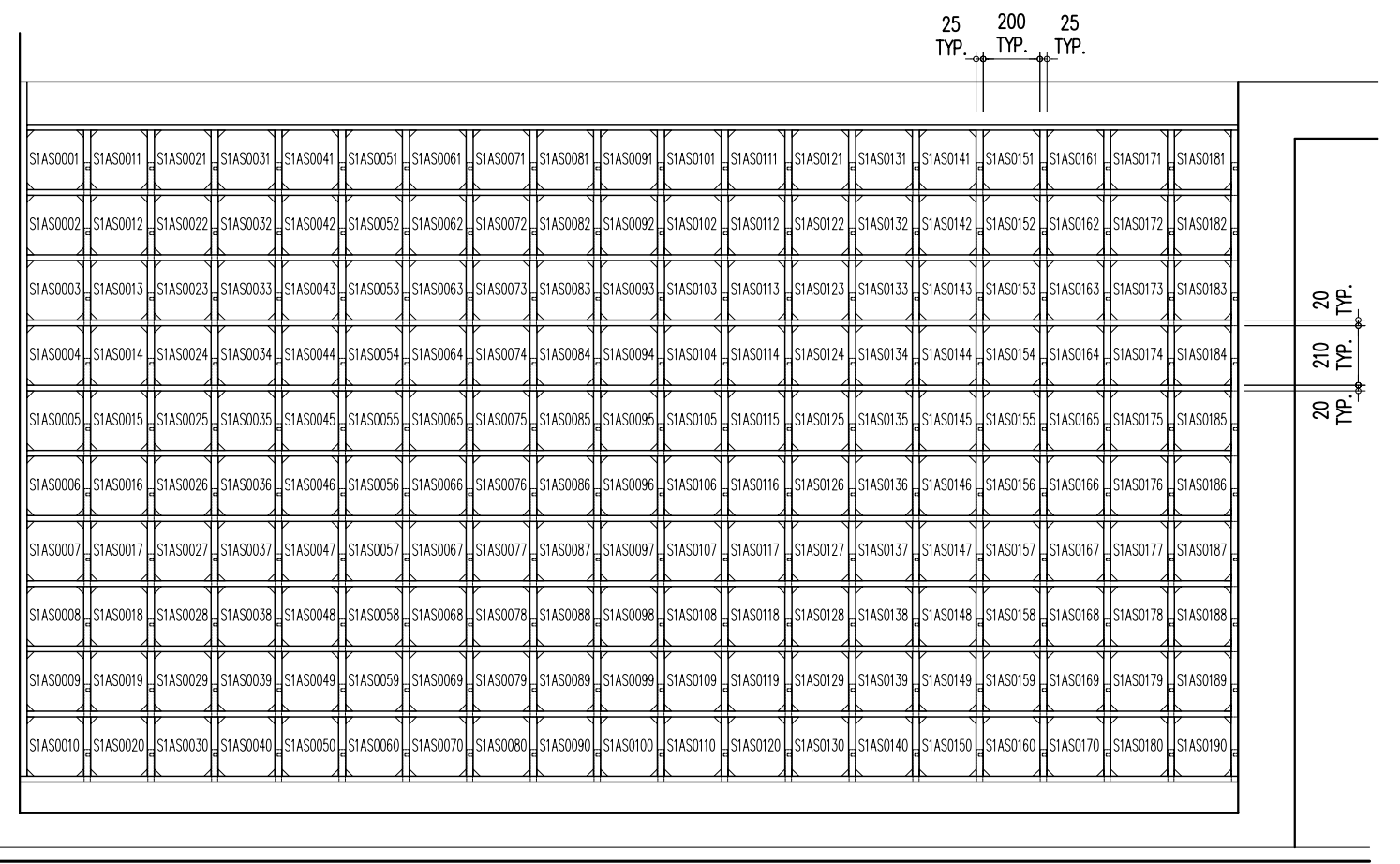
S1AS001 ~ S1AS0190 一樓立面圖 A
