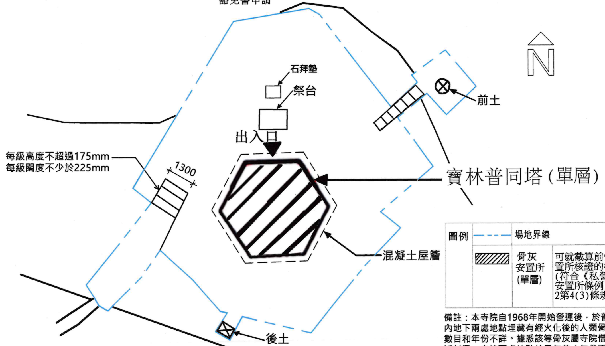
建議布局圖 (1:100) (圖則編號002) (按公制比例繪製)
