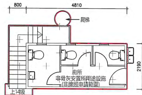
非骨灰安置所大樓地下樓面平面圖
