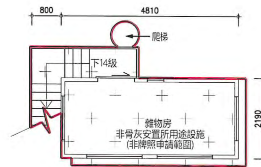
非骨灰安置所大樓一層樓面平面圖
