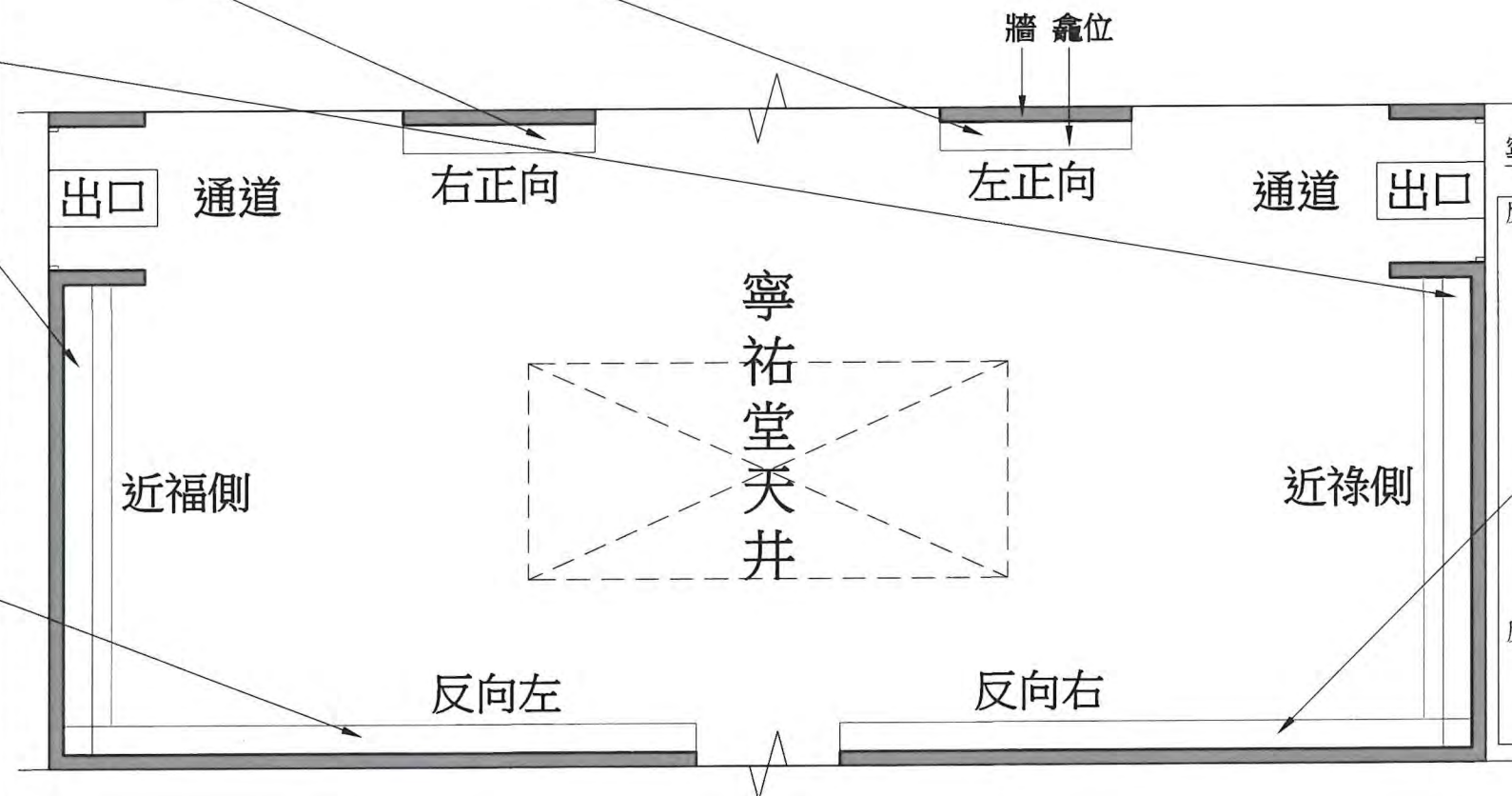
建議骨灰安置所大樓 3 (寧祐堂) - 地下 樓面平面圖 - (圖則編號 T3BD-3) 1:75 (按公制比例繪製)
