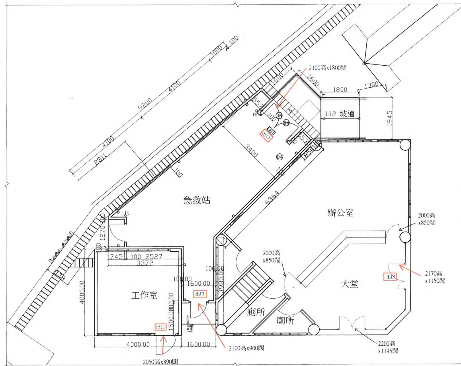
現有設施-急救站(地下) 樓面平面圖 - (圖則編號 FA1) 1:100 (按公制比例繪製)
