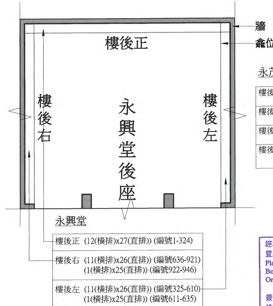
建議骨灰安置所大樓 1 (永興堂) - 一樓 樓面平面圖 - (圖則編號 T1BD-7) 1:75 (按公制比例繪製)
