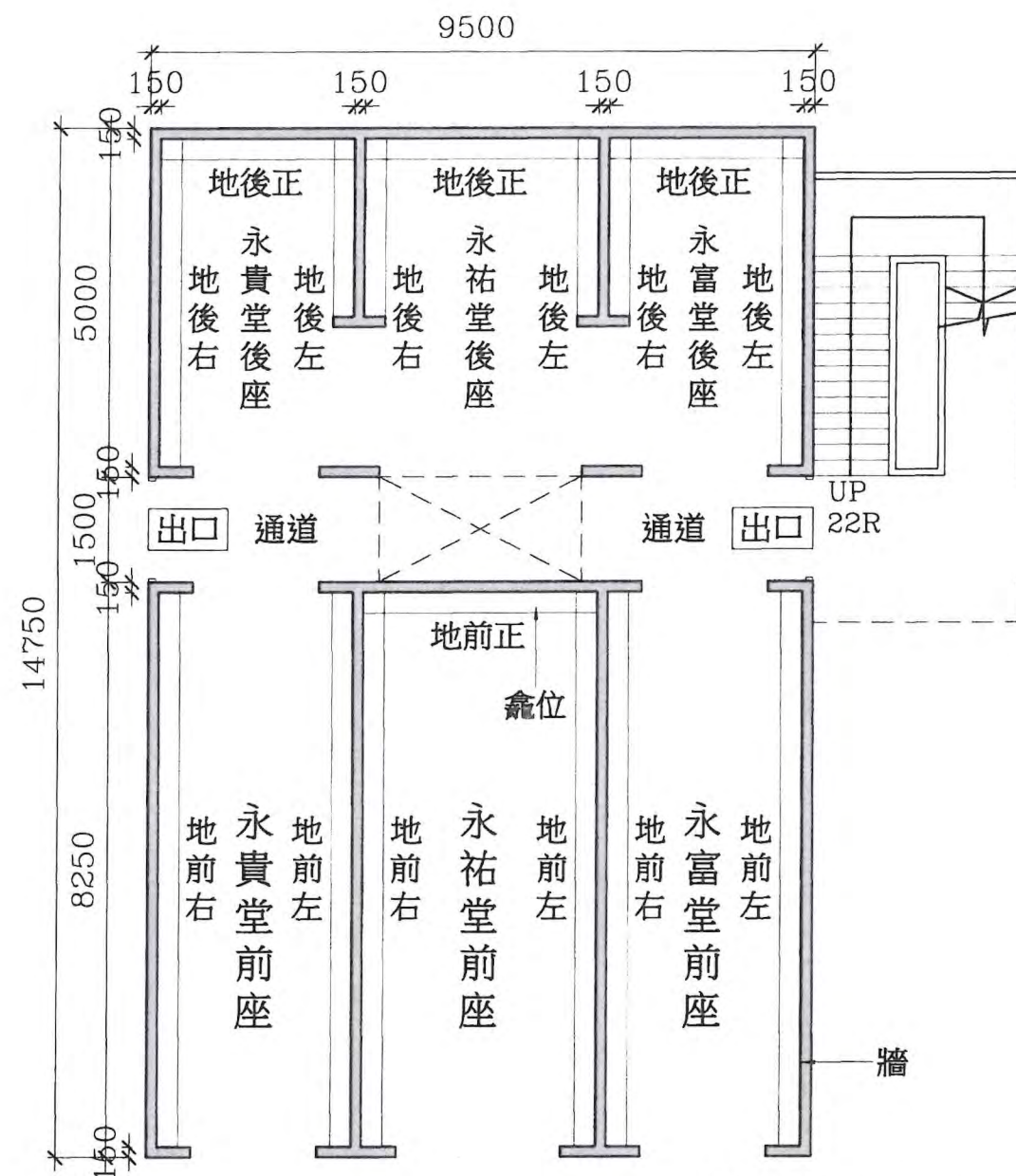
骨灰安置所大樓 6 地下 建築面積: 131.425 平方米
