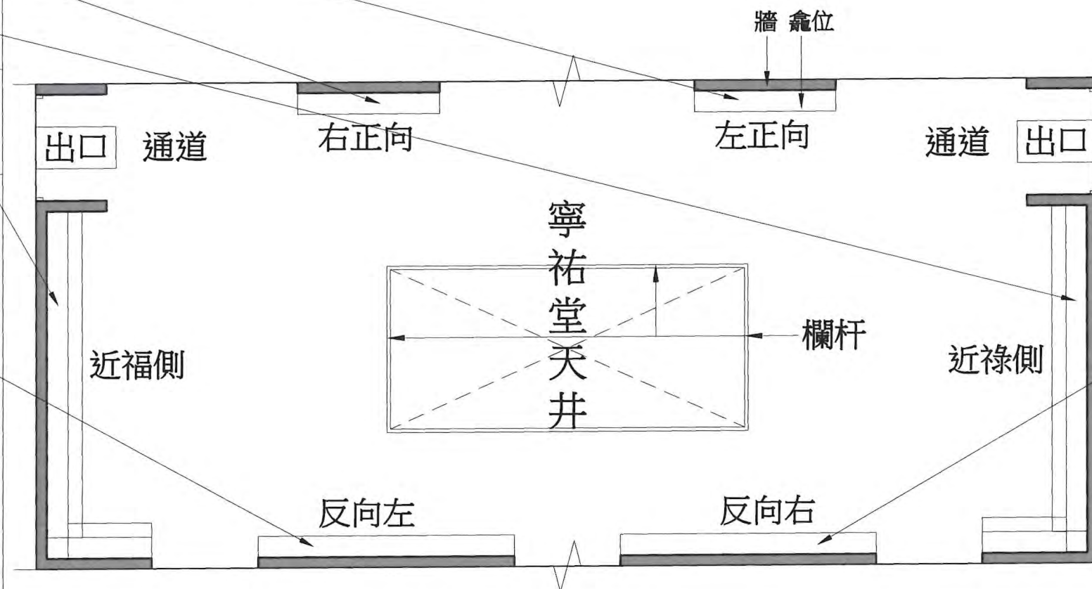
建議骨灰安置所大樓 3 (寧祐堂) - 一樓 樓面平面圖 - (圖則編號 T3BD-4) 1:75 (按公制比例繪製)
