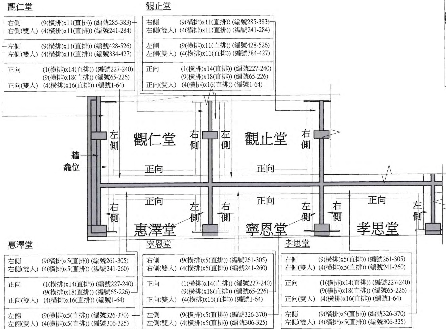
建議骨灰安置所大樓7(寧安樓) - 地下 樓面平面圖 - (圖則編號 T7BD-34) 1:75 (按公制比例繪製)
