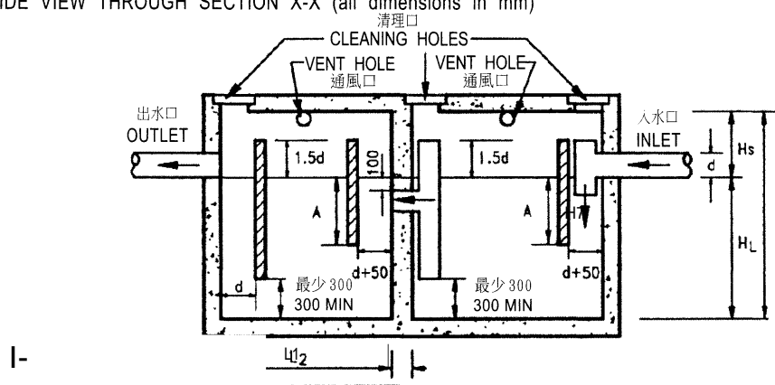
橫切面 X-X 側視圖（尺寸均以毫米為單位） SIDE VIEW THROUGH SECTION X-X (all dimensions in mm)
