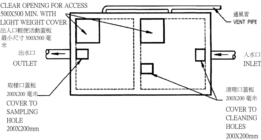
隔油池頂部外視圖（尺寸均以毫米為單位） EXTERNAL TOP VIEW OF GREASE TRAP (all dimensions in mm)
