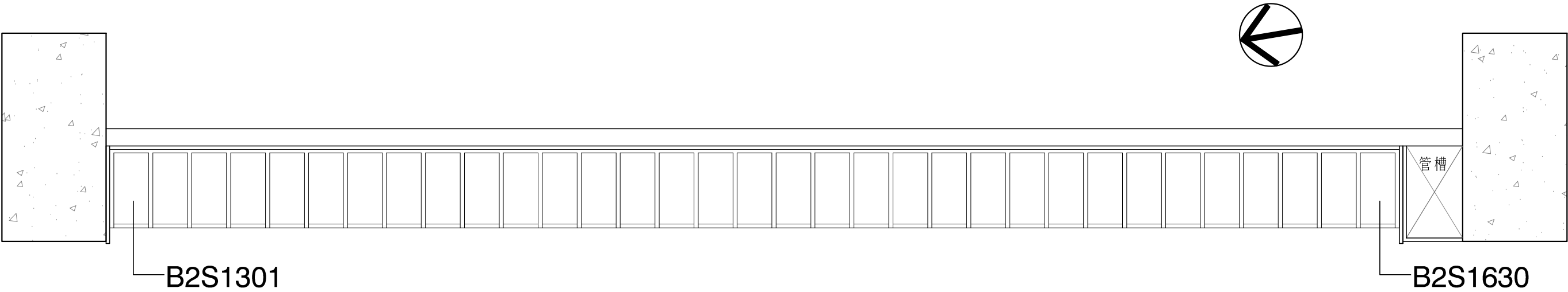
二樓平面圖5 Second Floor Plan Map 5
