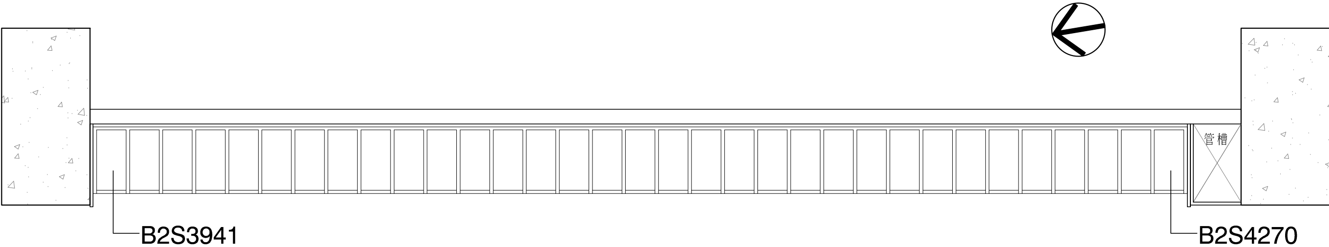
二樓平面圖13 Second Floor Plan Map 13
