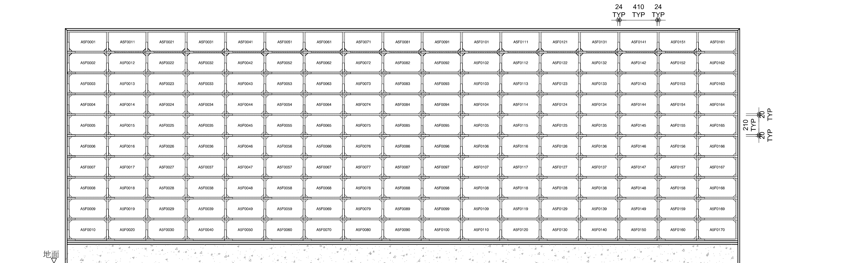
A5F0001 ~ A5F0170 五樓立面圖68
