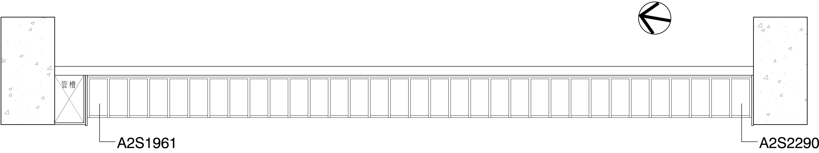
二樓平面圖7
