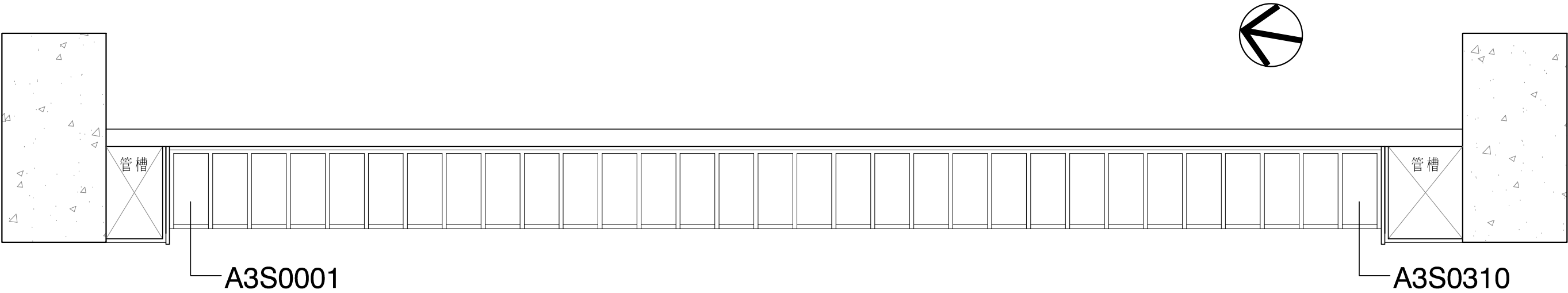
三樓平面圖19
