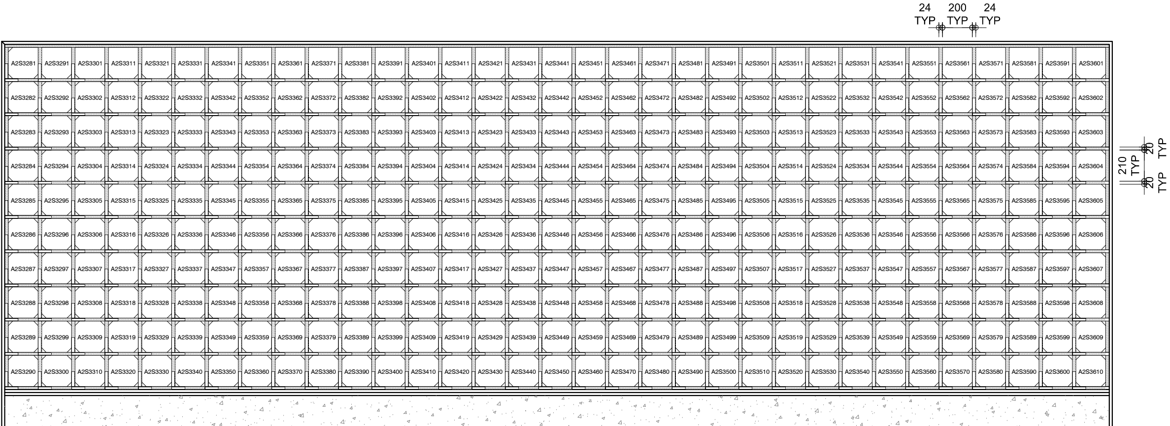
A2S3281 ~ A2S3610 二樓立面圖11
