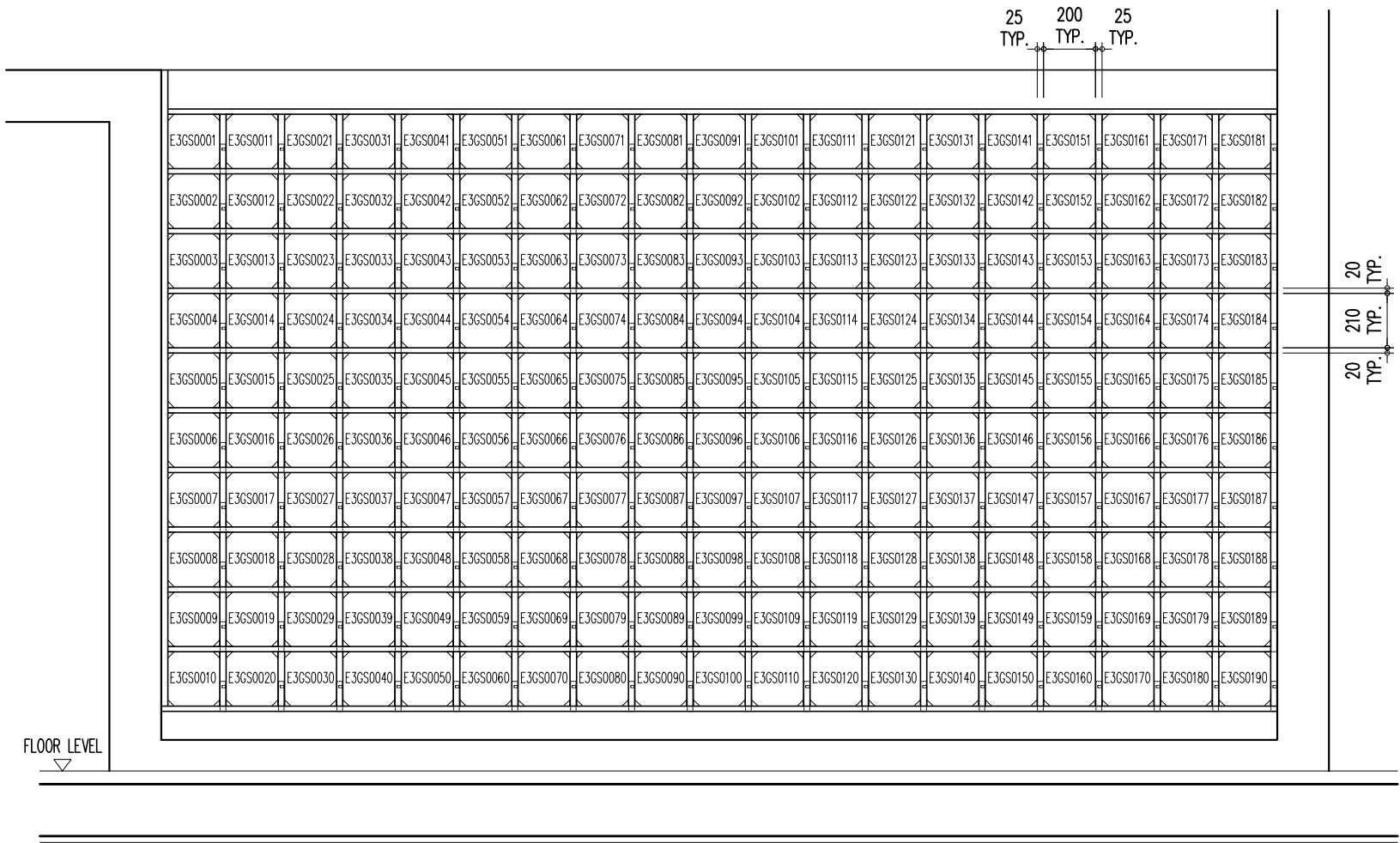
E3GS0001 ~ E3GS0190 3/F ELEVATION A
