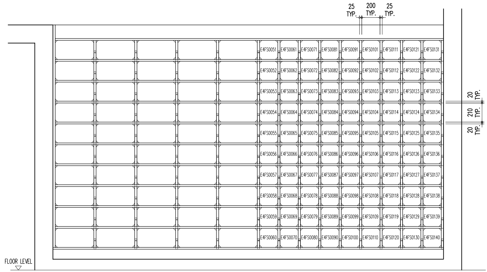
E4FS0051 ~ E4FS0140 4/F ELEVATION A
