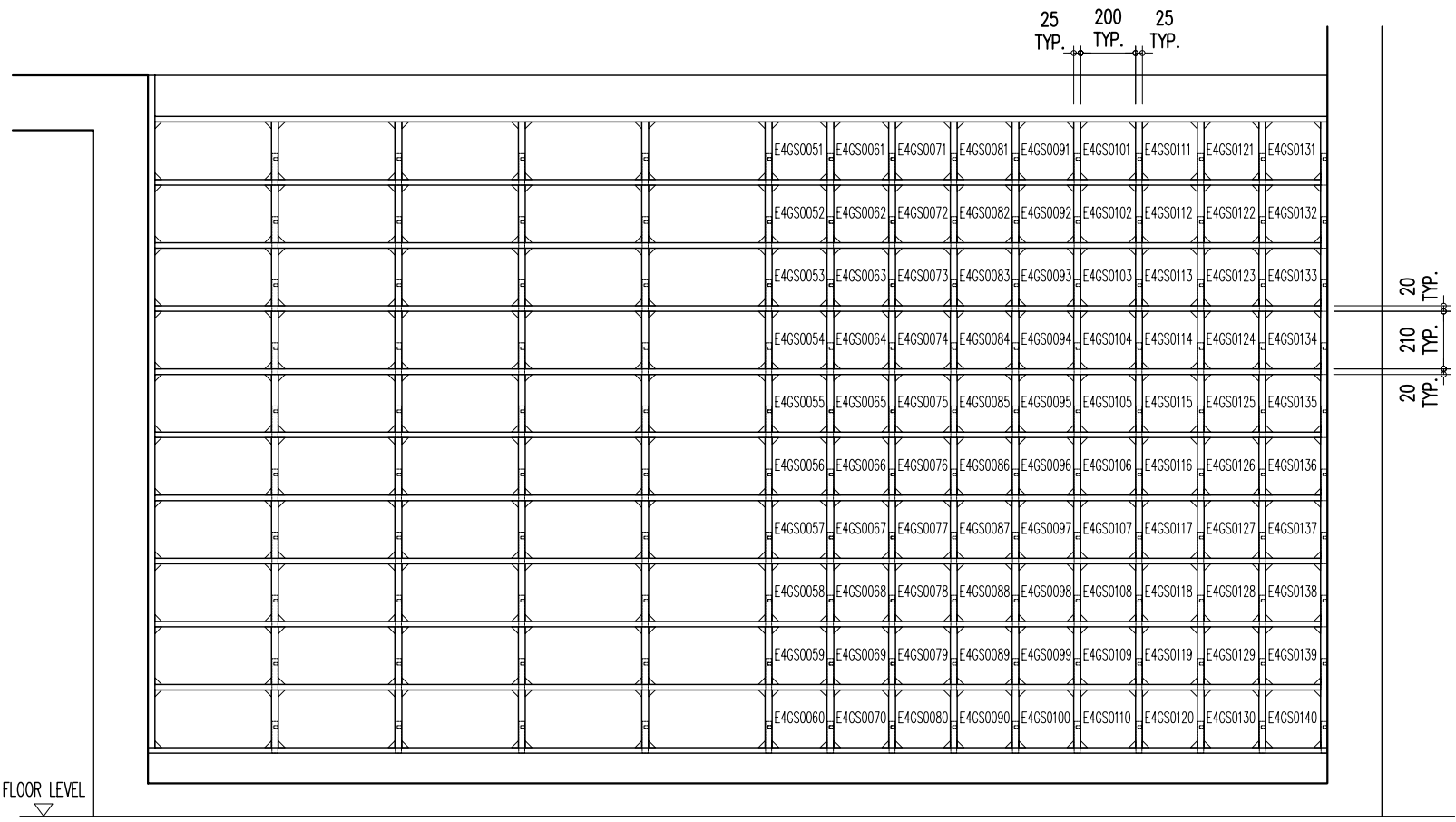
E4GS0051 ~ E4GS0140 4/F ELEVATION A
