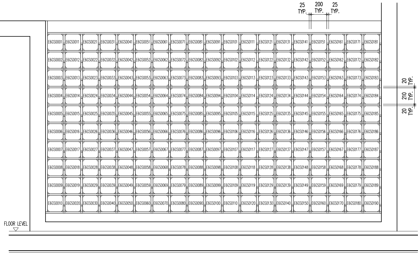
E6GS0001~ E6GS0190 6/F ELEVATION A
