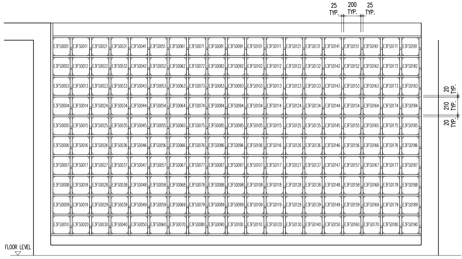
E3FS0001 ~ E3FS0190 3/F ELEVATION A
