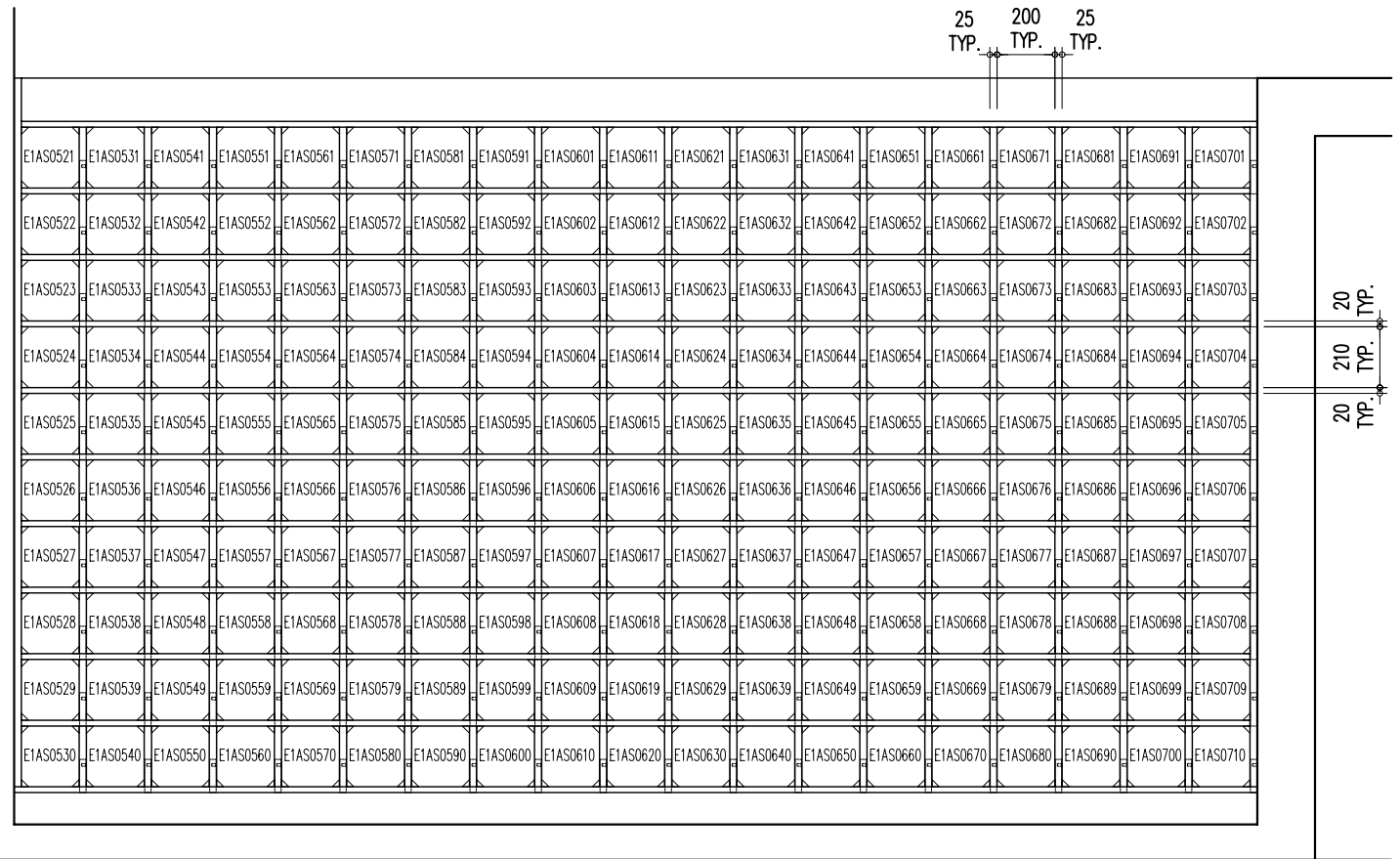
E1AS0521 ~ E1AS0710 1/F ELEVATION A
