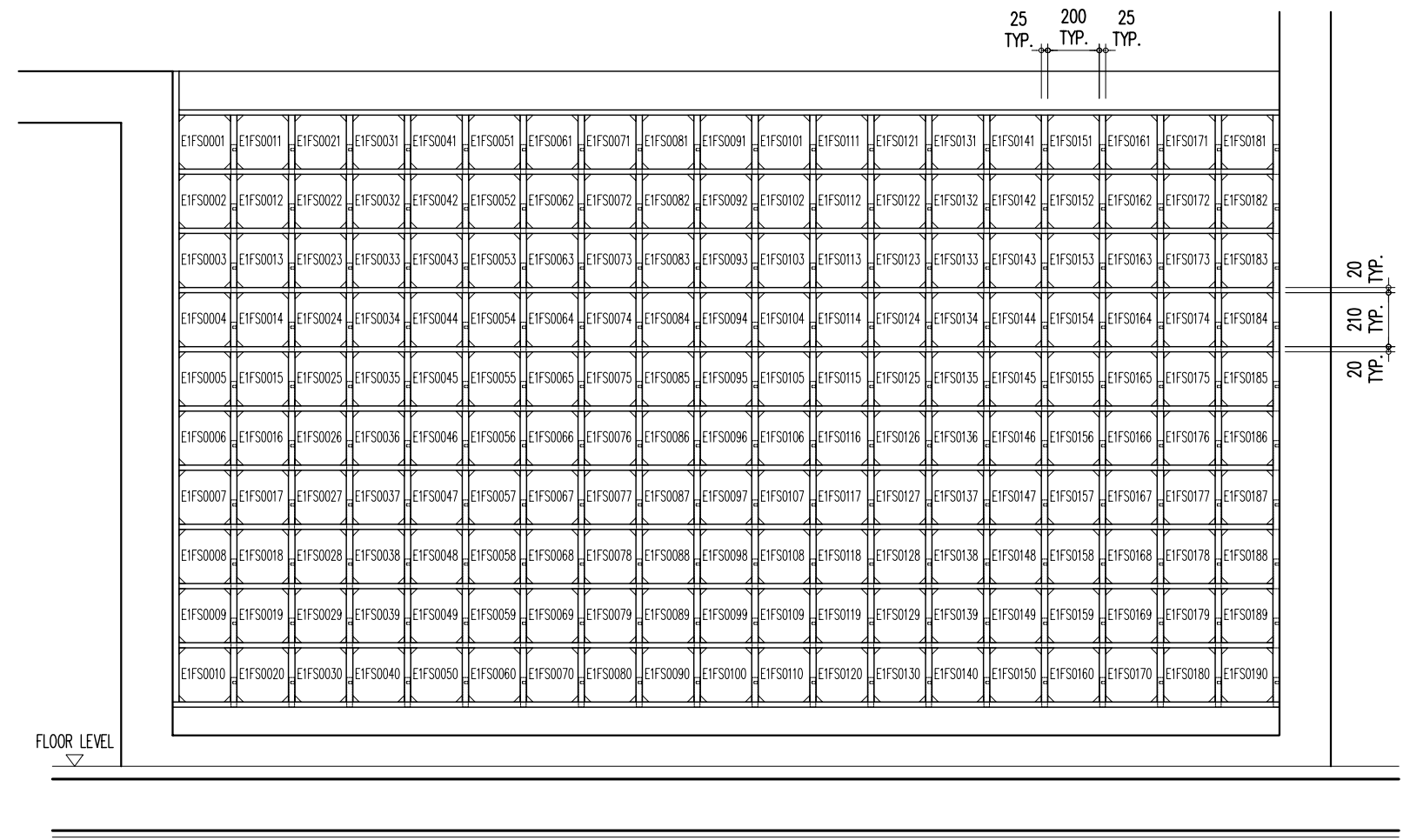
E1FS0001 ~ E1FS0190 1/F ELEVATION A
