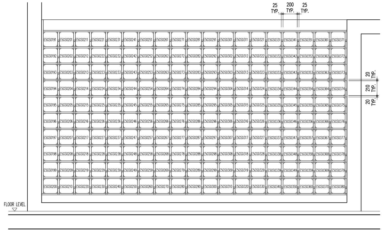
E5GS0191~ E5GS0380 5/F ELEVATION A
